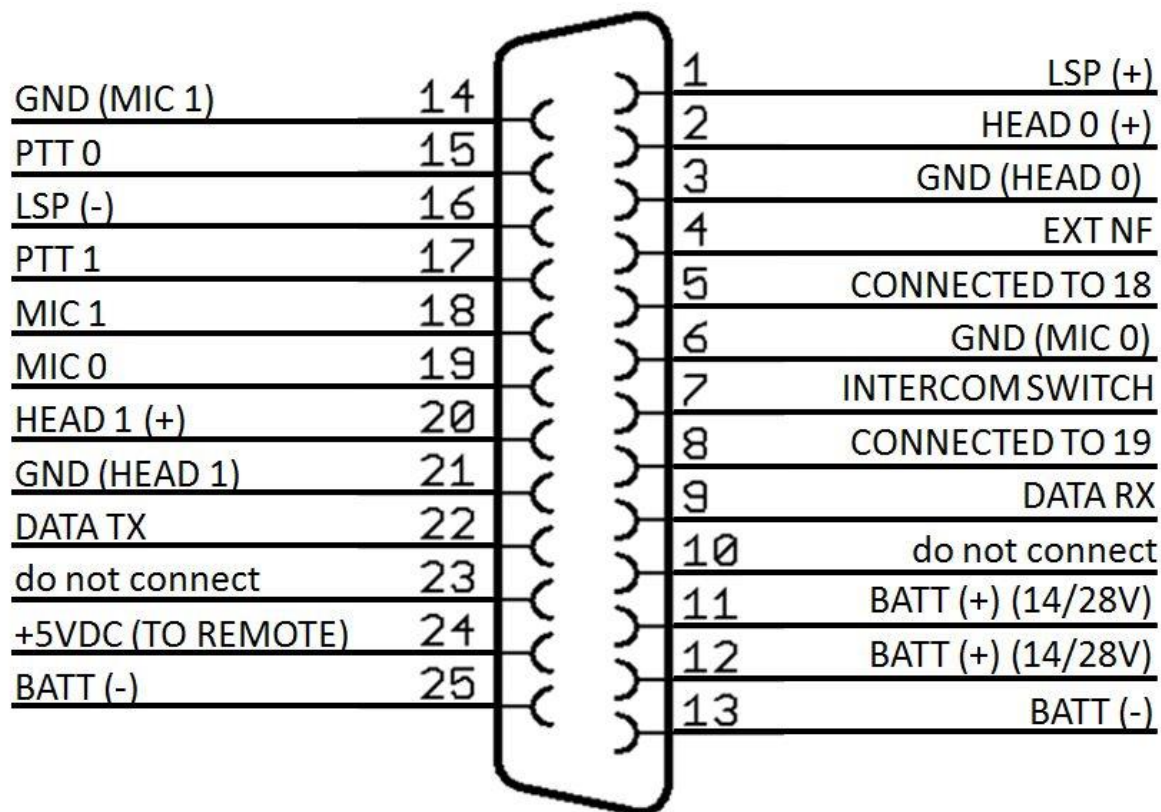
25-poliger Anschlussstecker am ATR833-II Ansicht von flugzeugseitiger Bestückungsseite
